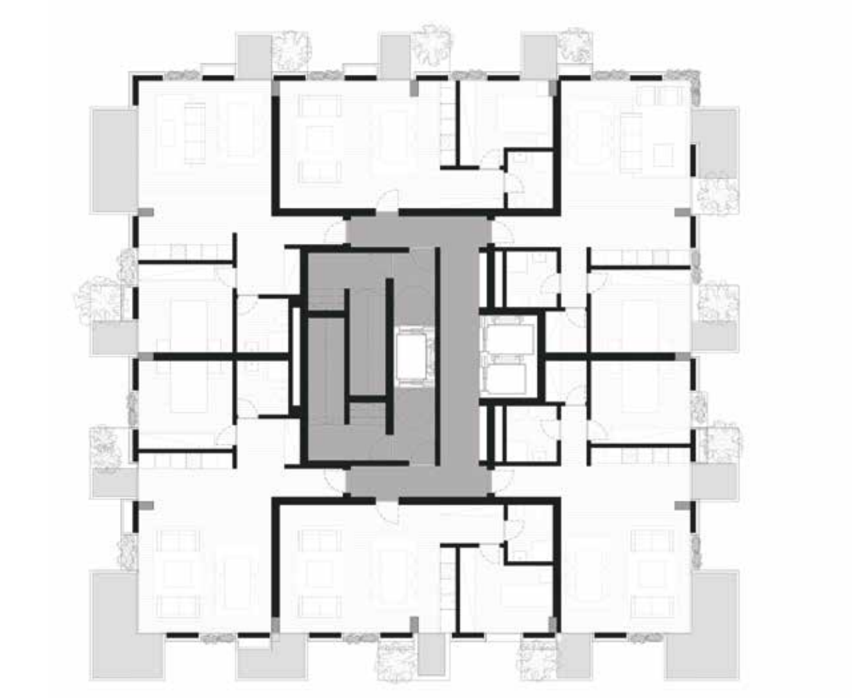
Planta tipo / Standard floor
